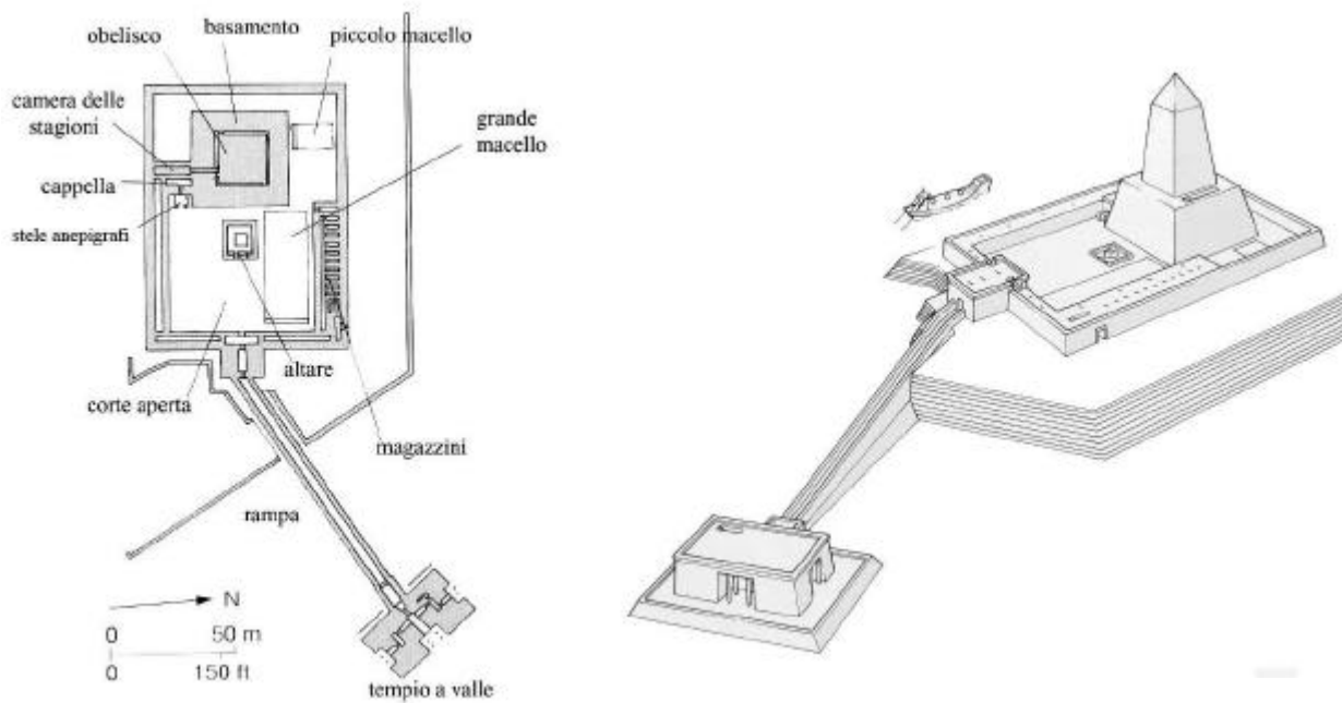
Figura 3. Pianta (sinistra) e ricostruzione (destra) del tempio solare di Niuserra. Disegno di Lehner dall'originale di Borchartd.
