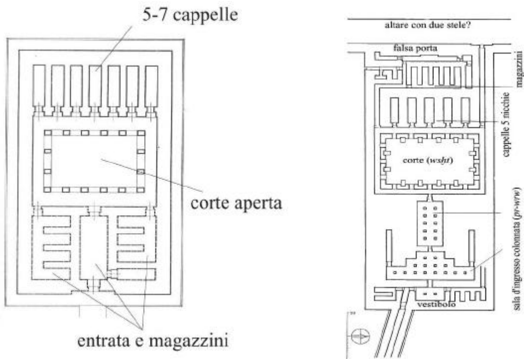
Figura 0. Pianta del tempio a valle del tempio solare di Userkaf (sinistra) e del tempio funerario della piramide di Khafra (destra).
